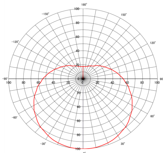
[配光特性] (1/2配光角 190°)
